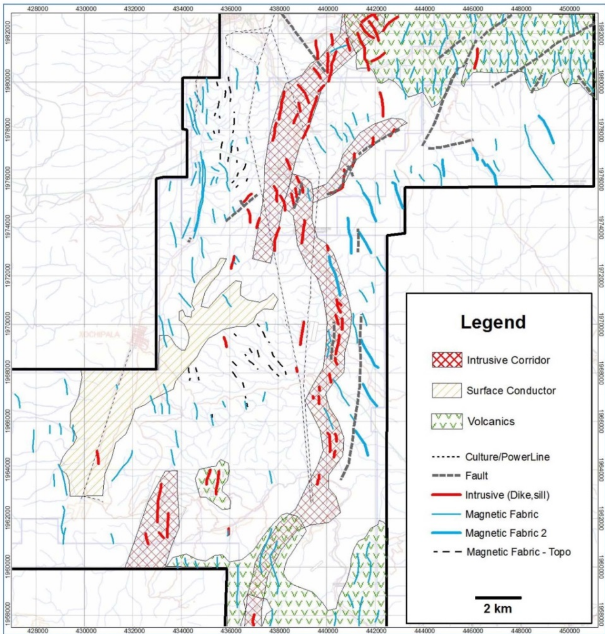
Figure 28 Mag interpretation
